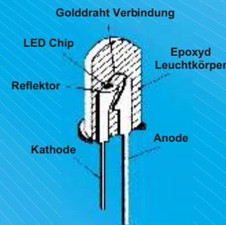
Bestandteile einer LED
