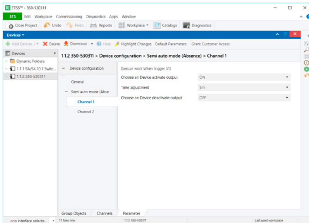
Abbildung 7: Halbautomatikmodus – Kanal 1
