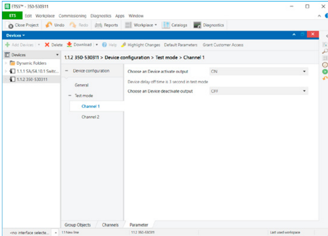
Abbildung 8: Testmodus – Kanal 1
