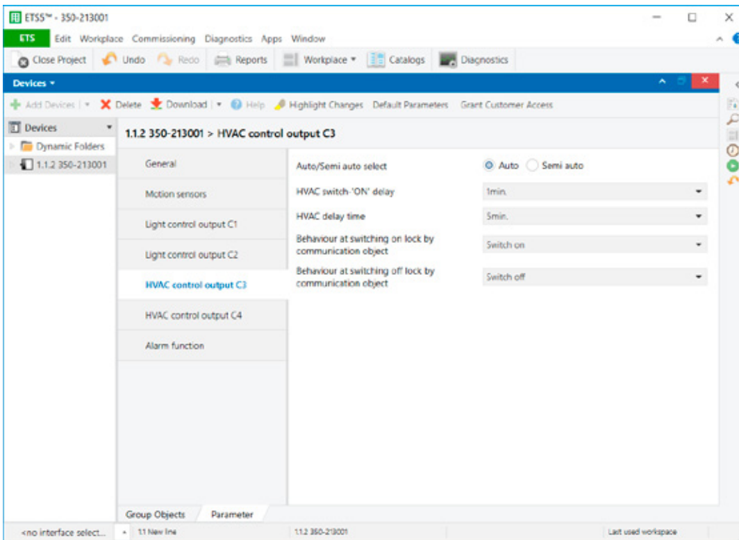
Abbildung 6: HLK-Steuerungsausgang
