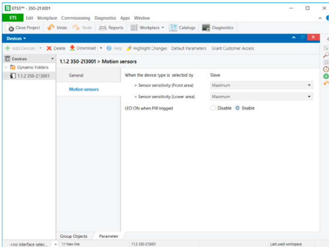
Abbildung 4: Bewegungssensoren – Slave
