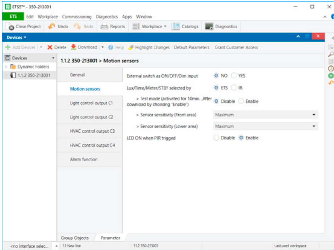
Abbildung 3: Bewegungssensoren – Master
