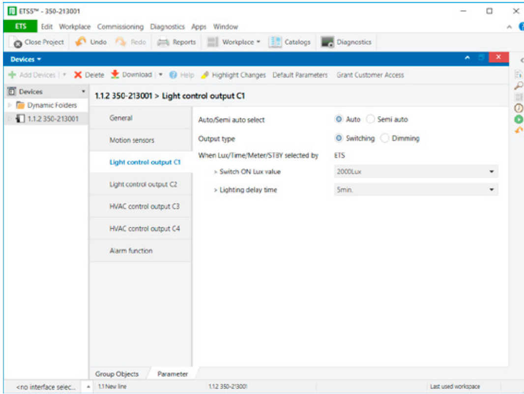
Abbildung 4: Lichtsteuerungsausgang – Schalten
