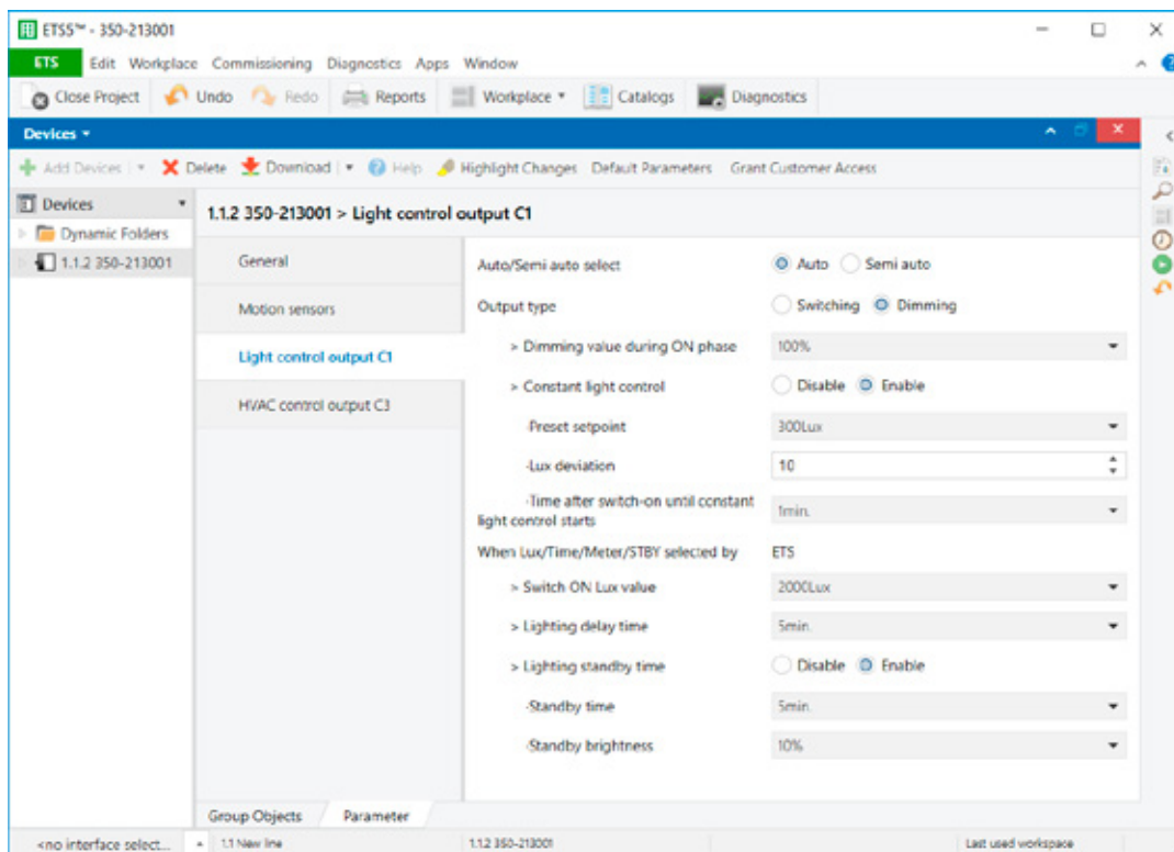
Abbildung 5: Lichtsteuerungsausgang – Dimmen
