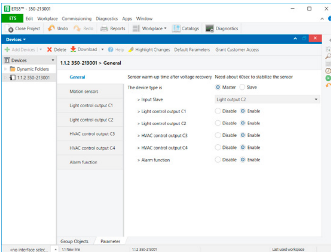
Abbildung 2: Allgemeines Panel
